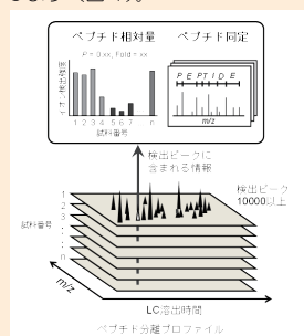
図 1. 非標識 (Label-free) LC-MS/MS の原理
